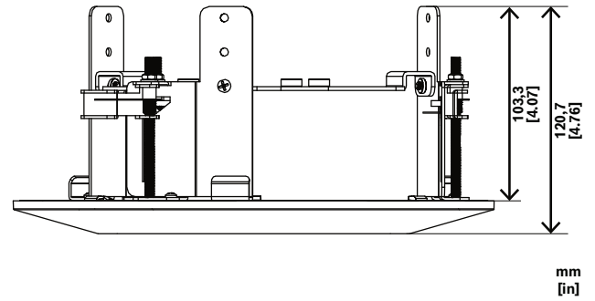
Şek. 1: NDA-8002-IC Kızılötesi
