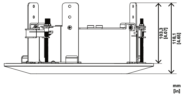
Şek. 2: NDA-8002-IC Kızılötesi Olmayan mm (inç) olarak boyutlar
